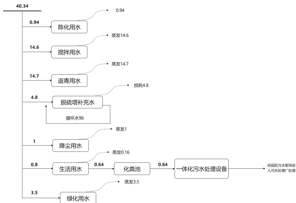
图 2-2 项目水平衡图（远期） 单位（m³/d）
