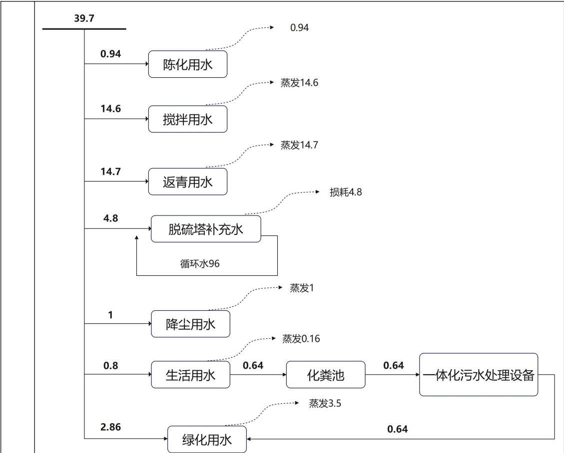
图 2-1 项目水平衡图（近期） 单位（m 3 /d）
