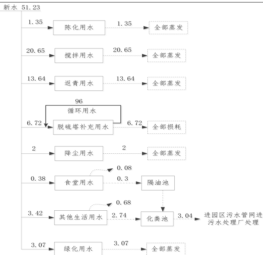
图 2-2 项目水平衡图（远期） 单位：m³/d
