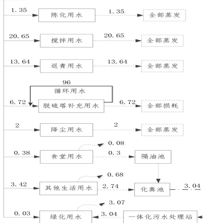
图 2-1 项目水平衡图 (近期) 单位: m 3 /d
